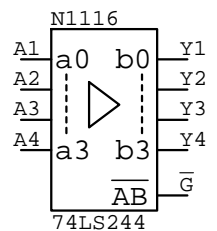
74LS244
