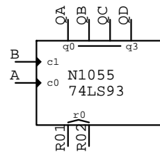
74LS93
