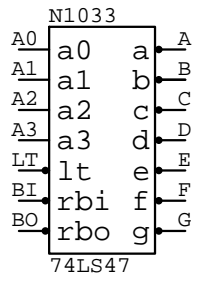
74LS47 N?????
