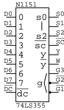
74LS355 N????
