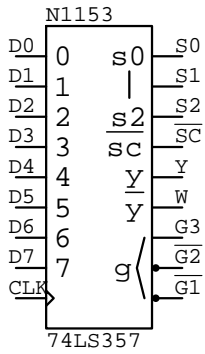
74LS357 N????
