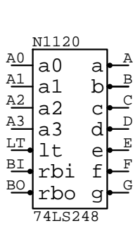
74LS248 N????
