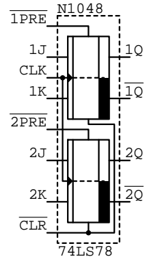
74LS78
