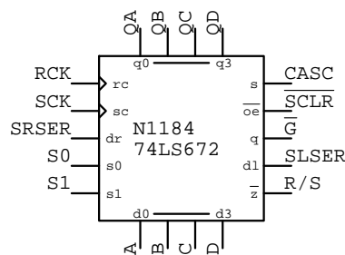
74LS672
