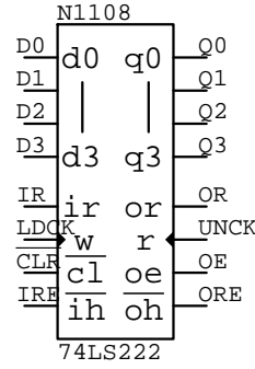
74LS222
