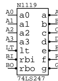
74LS247
