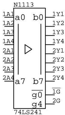
74LS241
