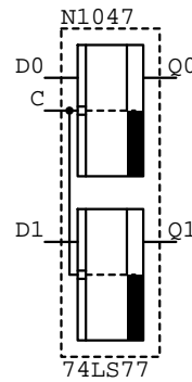
74LS77
