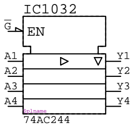
74AC244
