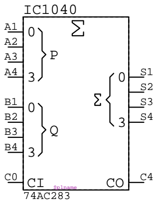
74AC283
