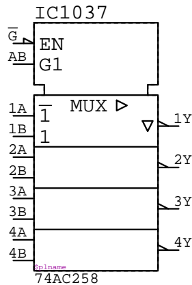
74AC258
