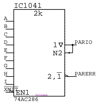
74AC286
