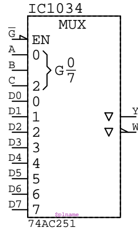
74AC251
