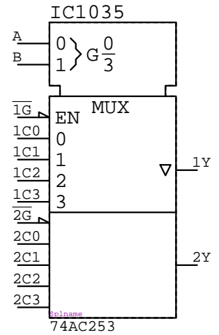
74AC253
