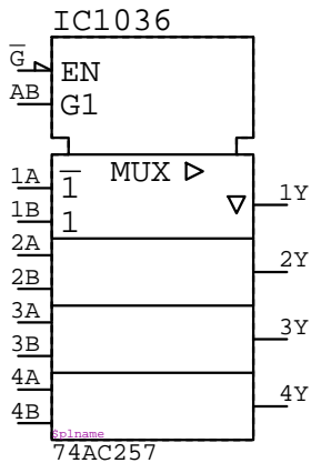
74AC257
