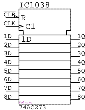
74AC273
