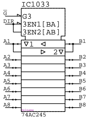
74AC245
