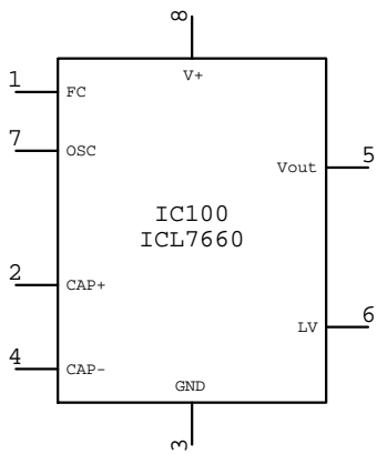
ICL7660 IC???
